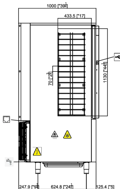
Vista Laterale Lateral side
