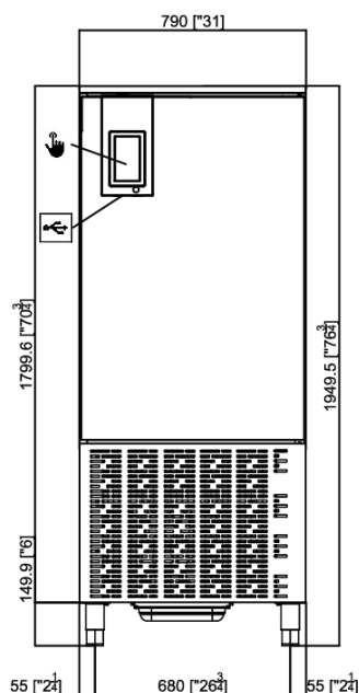
Vista Frontale Frontal side
