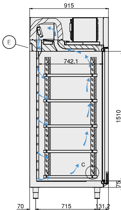
Sez. B-B
